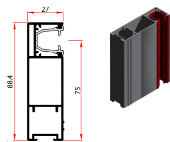
ALU vodilo sistema MODUL z možnostjo naknadne vgraditve integriranega rolo komarnika.
