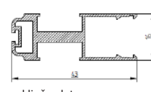
zaključna letva
