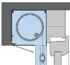
PODOMETNA MONTAŽA rolo omarica je skrita za fasado
