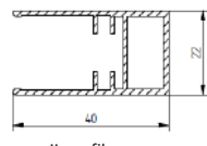
zgornji profil
