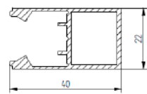
stranski profil
