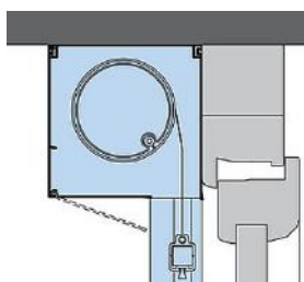
NADOMETNA MONTAŽA rolo omarica je vidna
