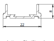
spodnji profil višine 8mm
